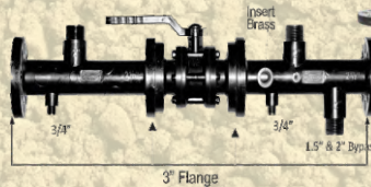
PP Header (2", 2.5", 3")
